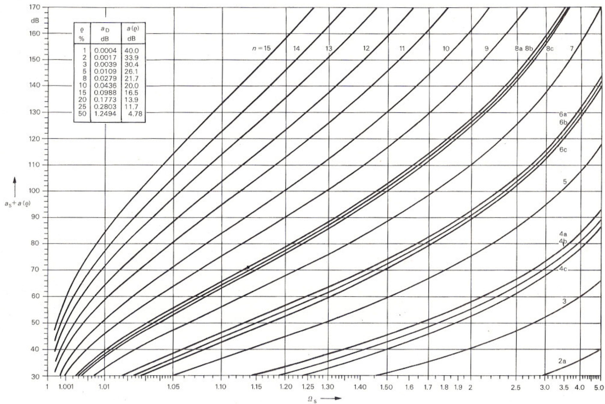
Bild 2.7 Diagramm zur Aufwandsabschätzung für Cauerparameter-Tiefpässe
